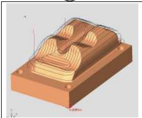
3D切削加工データ作成
